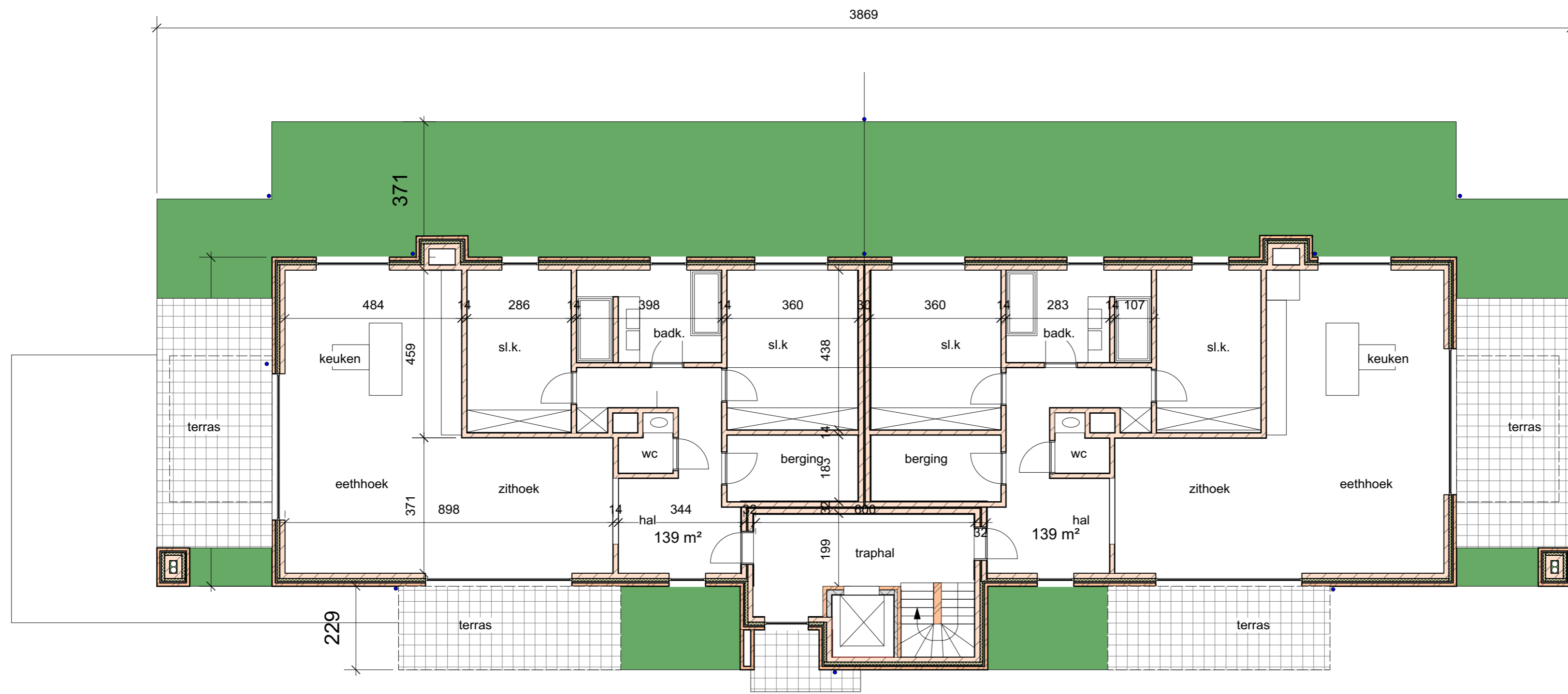
DAKVERDIEPING 1/100
