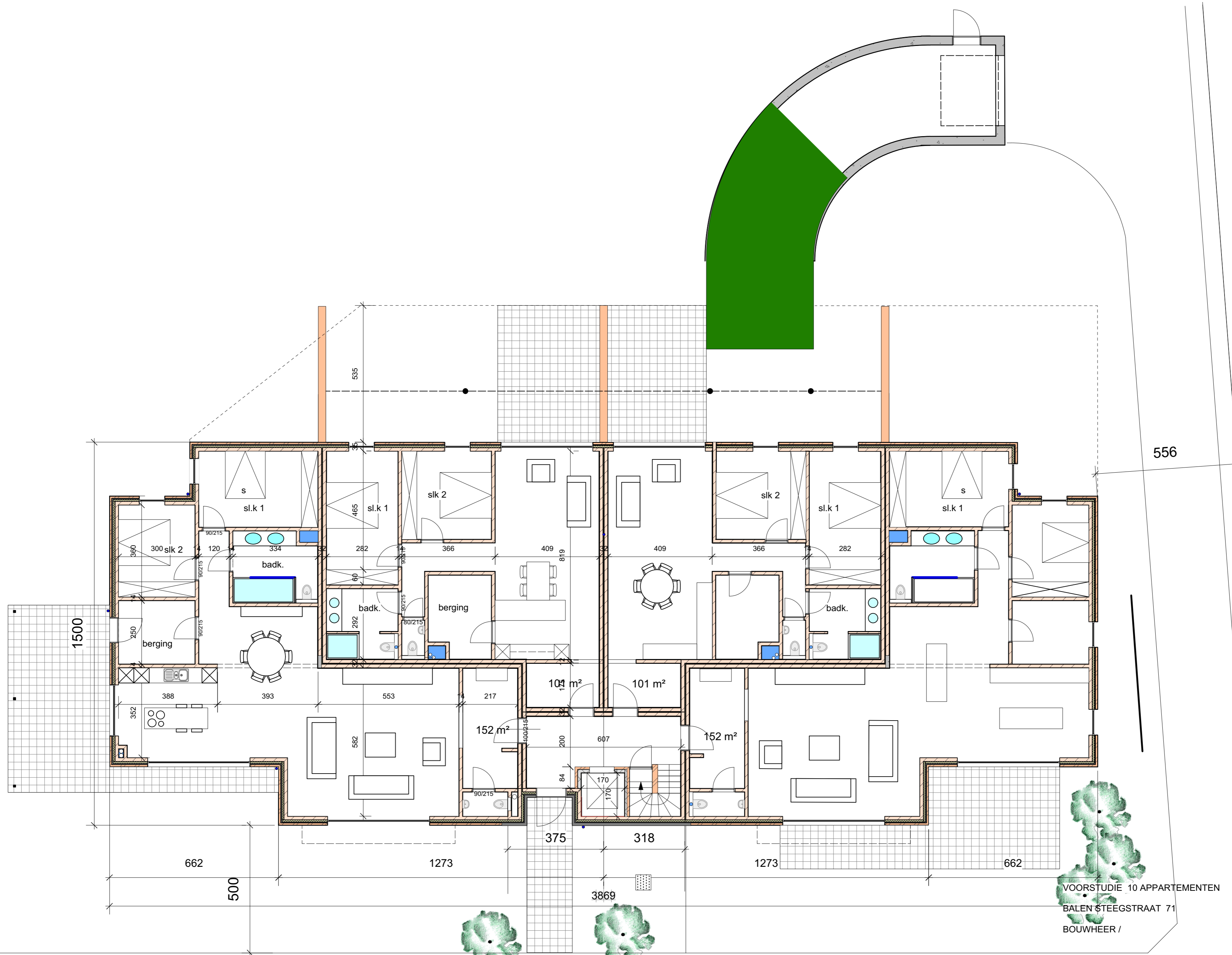
GELIJKVLOERS 1/100
