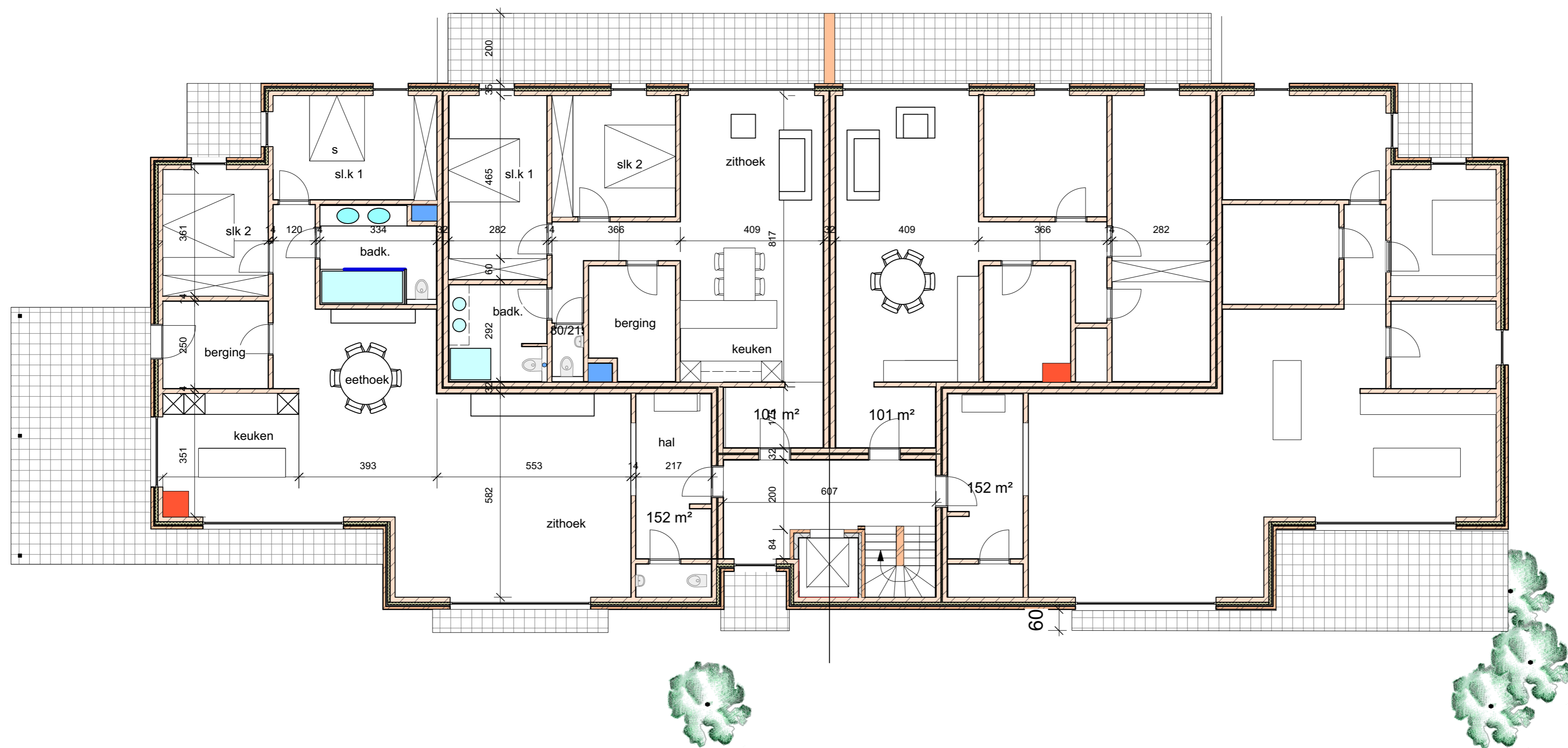
EERSTE VERDIEPING 1/100
